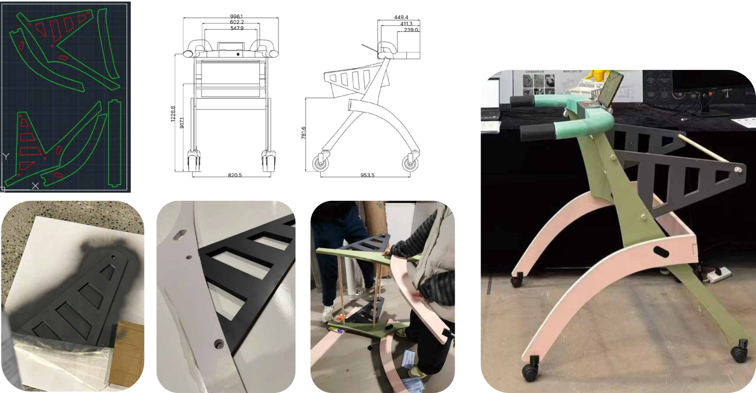
购物车设计1: 1模型（可正常推行）
